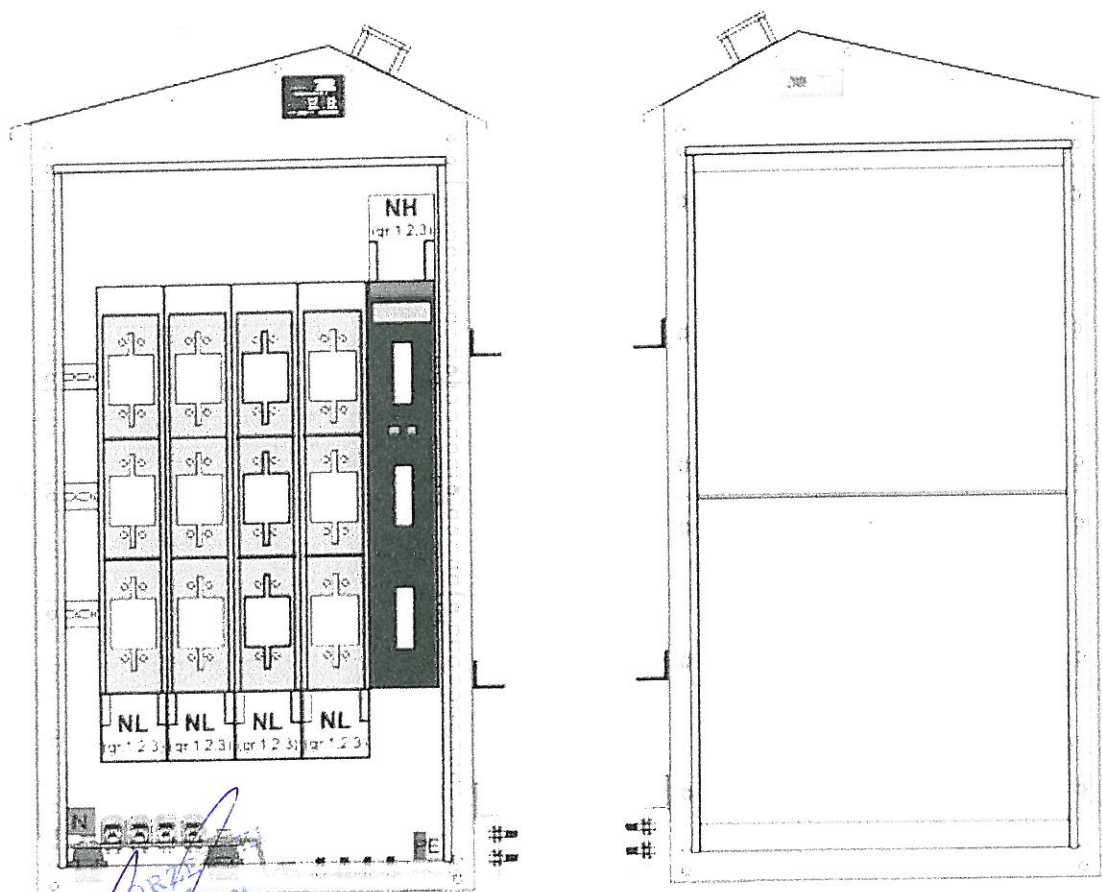
Schemat elektryczny
