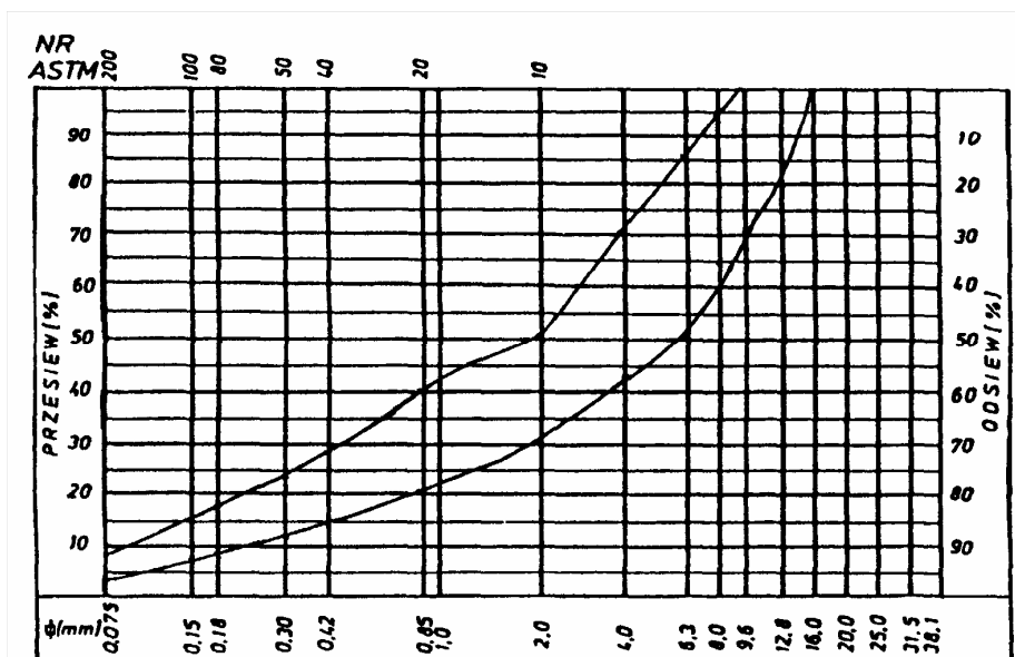
Rys. 9. Krzywe graniczne uziarnienia mieszanki mineralnej 0+16 mm do warstwy wiążącej, wyrównawczej z betonu asfaltowego dla KR 1-2
