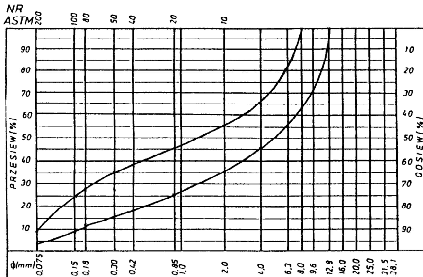
Rys. 10. Krzywe graniczne uziarnienia mieszanki mineralnej 0-12,8 mm do warstwy wiążącej, wyrównawczej z betonu asfaltowego dla KR 1-2
