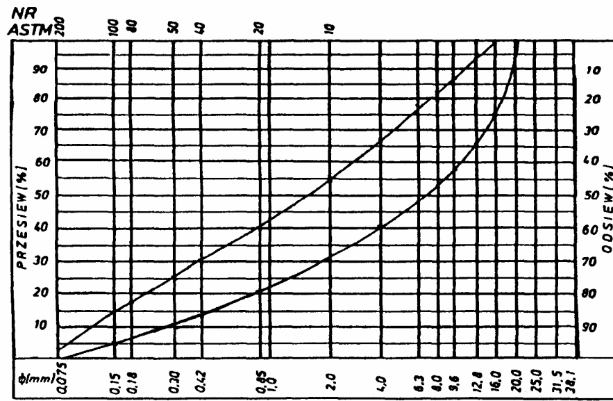
Rys. 8. Krzywe graniczne uziarnienia mieszanki mineralnej 0÷20 mm do warstwy wiążącej, wyrównawczej z betonu asfaltowego dla KR 1-2
