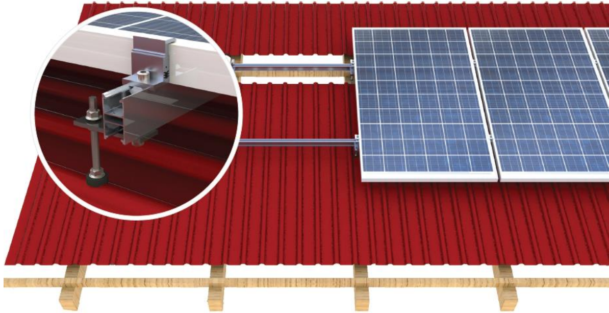
Rys. 9. Ilustracja przykładowego systemu montażu.
